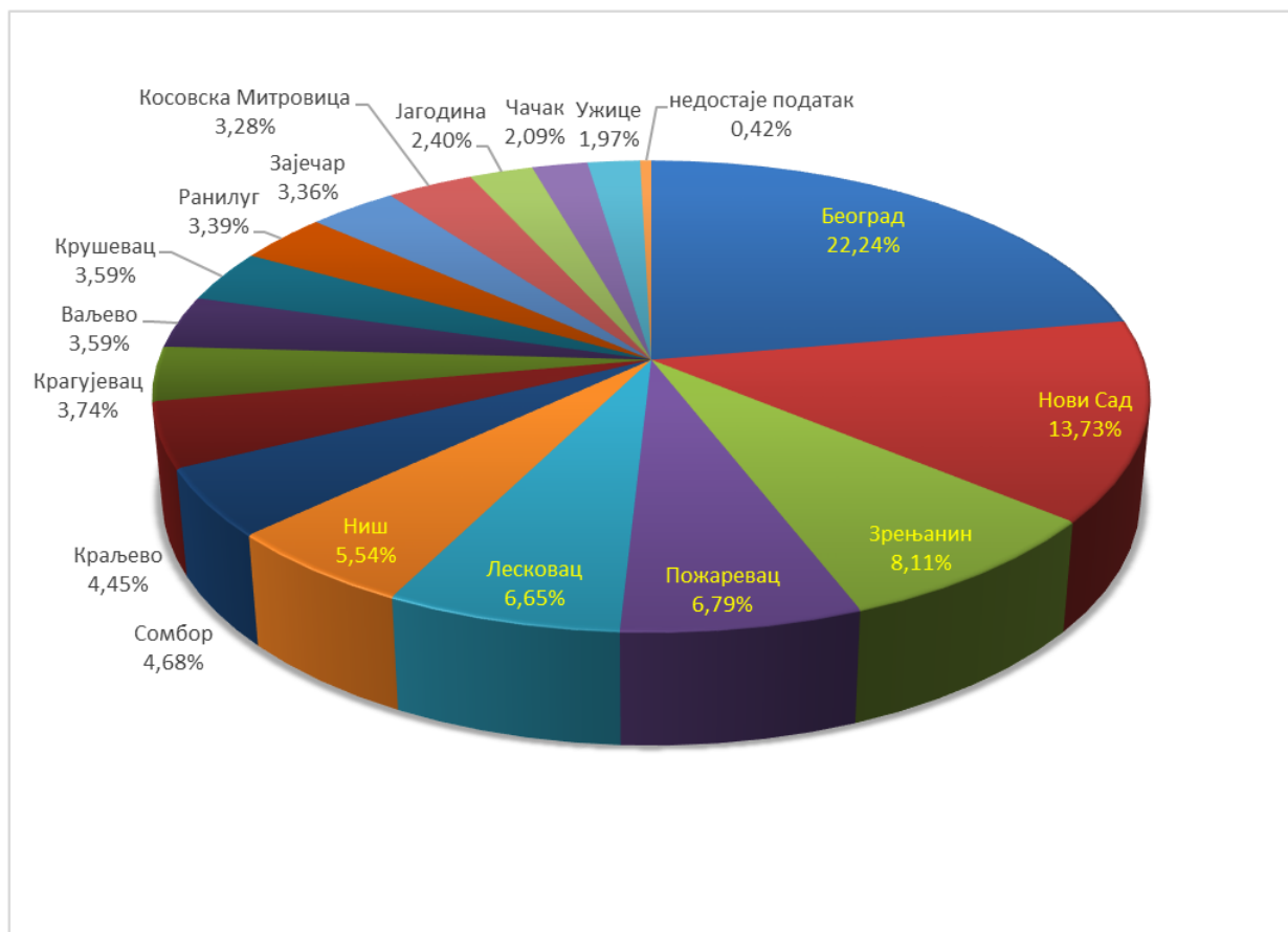
Процентуални однос број полазника по школској управи
